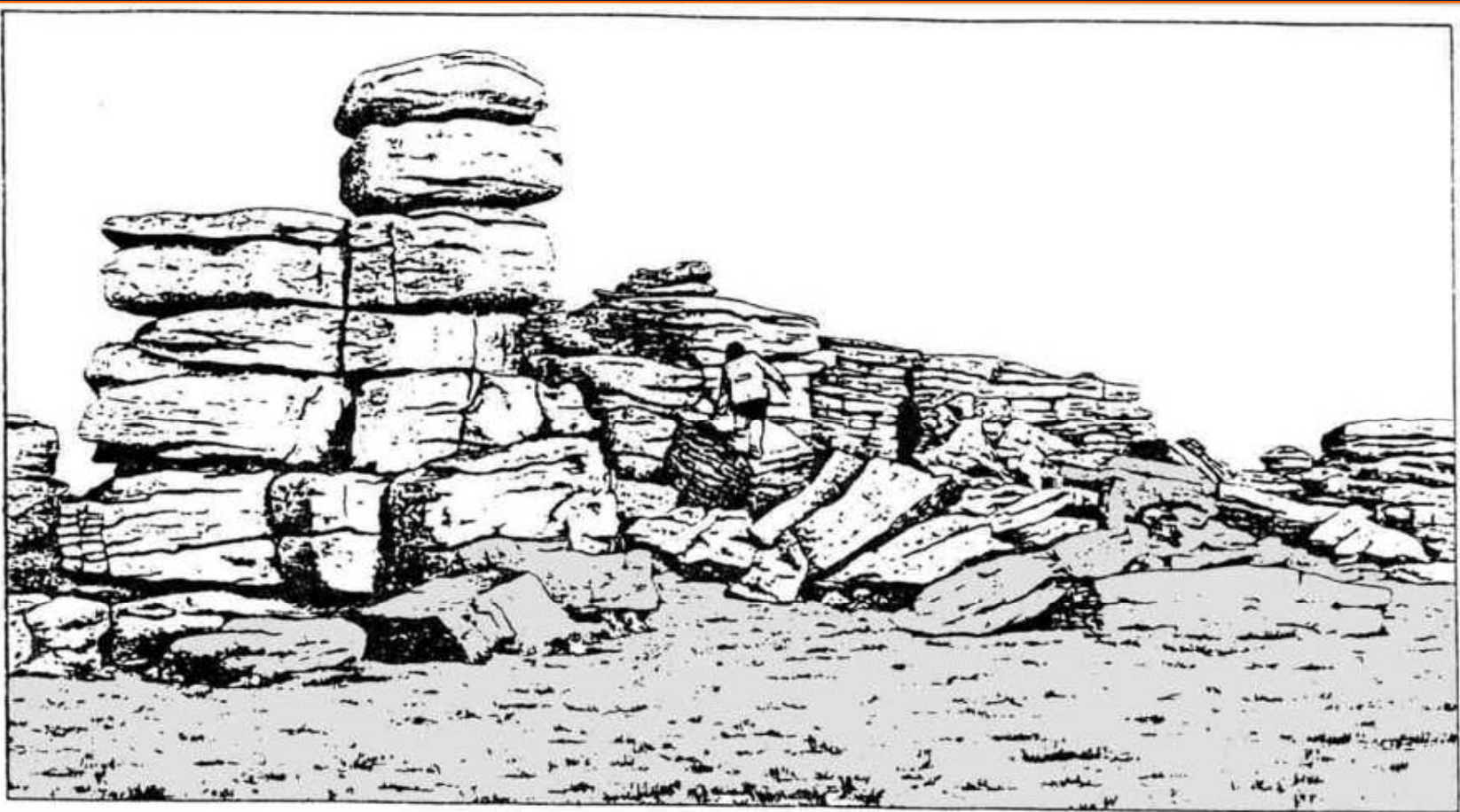
شکل ۳-۶. در اثر هوازدگی، گرانیت به صورت قطعات و بلوکهای متعددی درآمده است. درزها کاملاً باز شده‌اند و قطعات و بلوکها از هم جدا شده‌اند.
